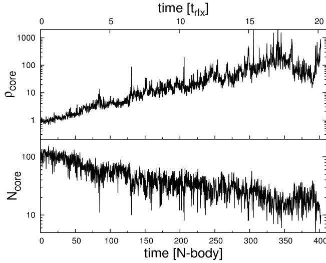
Σχήμα 6.27: Πυκνότητα μάζας στον πυρήνα (σε μονάδες N-σωμάτων) (επάνω διάγραμμα) και αριθμός αστέρων στον πυρήνα (κάτω διάγραμμα). Κατά τη στιγμή της κατάρρευσης του πυρήνα, η πυκνότητά του παίρνει μέγιστη τιμή.
