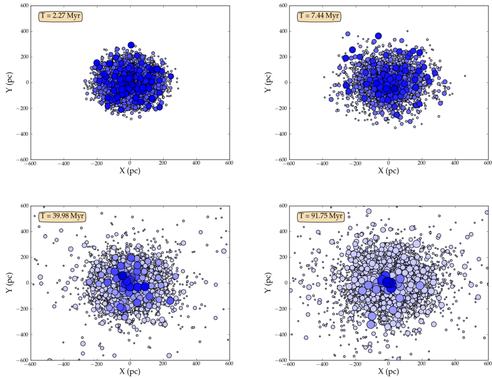
Σχήμα 7.21: Δημιουργία του “σπόρου” UCD στο κέντρο του CC. Προβολή όλων των αστρικών σμηνων στο επίπεδο X–Y για την προσομοίωση με κωδικό όνομα F3. Η ακτίνα των σμηνών έχει μεγεθυνθεί για λόγους παρουσίασης. Τα σμήνη με μεγαλύτερη μάζα παρουσιάζονται ως μεγαλύτερα σε μέγεθος και πιο σκούρα σε χρώμα σε σχέση με τα μικρότερα σμήνη κάθε εικόνας. Μετά από 7.44 Myr είναι φανερό πως τα μεγαλύτερα σε μάζα σμήνη δημιουργούνται κοντά στο κέντρο του CC. Αργότερα, σε χρόνο T \sim 40 \text{ Myr} όλα τα μεγαλύτερης μάζας σμήνη εντοπίζονται κοντά στο κέντρο του CC. Τέλος, στο τελευταίο σχήμα είναι φανερό πως υπάρχουν ορισμένα μεγάλα σμήνη κοντά στο κέντρο, στο οποίο βρίσκεται ένα πολύ μεγαλύτερο σμήνος. Η μάζα του σμήνους αυτού είναι 2.9 \times 10^6 M_{\odot} κανόντάς το να αποτελεί τον “σπόρο” από τον οποίο θα δημιουργηθεί εν τέλει ο UCD. Στην ηλεκτρονική διεύθυνση http://www.aei.mpg.de/~rau/6k_r248_rblue.ogg παρουσιάζεται ένα βίντεο της διαδικασίας.
