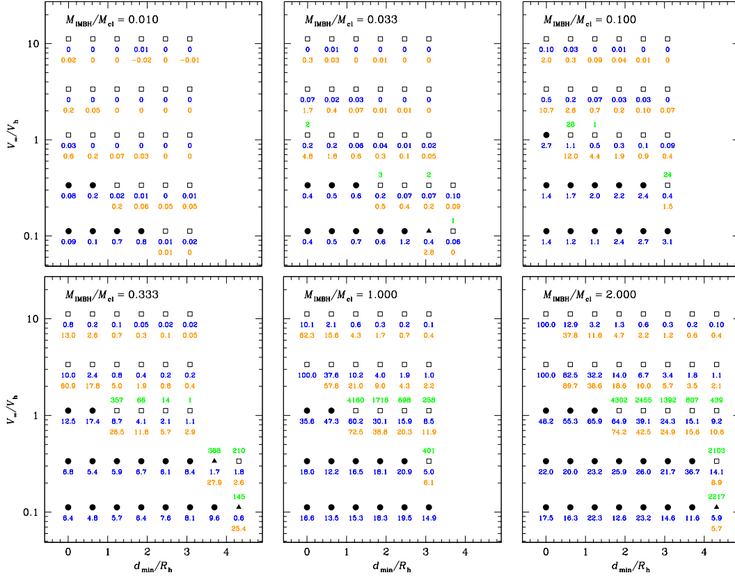
Σχήμα 7.17: Αποτελέσματα των 196 προσομοιώσεων της διέλευσης μιας IMBH μέσα από ένα σμήνος αστέρων με παράμετρο King W_0 = 7 . Κάθε πάνελ δείχνει τα αποτελέσματα για μια συγκεκριμένη τιμή του λόγου μαζών M_{\bullet}/M_{cl} . Ο x-άξονας σε κάθε σχήμα είναι η απόσταση d_{min} , σε μονάδες της ακτίνας μισής μάζας R_h του σμήνους. Ο y-άξονας είναι η σχετική ταχύτητα στο άπειρο των δύο σωμάτων, σε μονάδες της ταχύτητας διασποράς V_h \equiv (GM_{cl}/R_h)^{1/2} του σμήνους. Οι “γεμάτες” τελείες υποδεικνύουν “συγκρούσεις” δηλαδή περιπτώσεις στις οποίες η IMBH παγιδεύτηκε από το σμήνος και κατέληξε στο κέντρο του. Τα “γεμάτα” τρίγωνα υποδεικνύουν περιπτώσεις όπου η IMBH παγιδεύτηκε σε τροχιά γύρω από το σμήνος αποτελώντας δορυφόρο του. Το τελικό αποτέλεσμα των περιπτώσεων αυτών αναμένεται να είναι επίσης σύγκρουση. Τα “Ανοιχτά” τετράγωνα αναφέρονται σε προσομοιώσεις στις οποίες η IMBH διαπέρασε το σμήνος χωρίς να παγιδευτεί στο βαρυτικό του πεδίο. Ο μπλε αριθμός ακριβώς από κάτω από κάθε σύμβολο, δείχνει το ποσοστό απώλειας μάζας του σμήνους. Ο δεύτερος ακριβώς από κάτω αριθμός, σε πορτοκαλί χρώμα, δείχνει το ποσοστό της μείωσης της ενέργειας σύνδεσης των δύο σωμάτων. Ο αριθμός ακριβώς από επάνω από το κάθε σύμβολο, υποδεικνύει τον αριθμό των αστέρων του σμήνους που έχουν παγιδευτεί από το βαρυτικό πεδίο της IMBH, στις περιπτώσεις που αυτή δεν έχει καταλήξει στο κέντρο του σμήνους.
