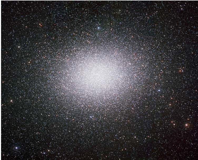
Σχήμα 2.1: Το σφαιρωτό σμήνος \omega -Centauri όπως παρατηρήθηκε από το ESO. Το απόλυτο οπτικό μέγεθος του είναι M_v = 10.4 , ενώ η ακτίνα μισού φωτός r_h \sim 2,79 \text{ arcmin} . Υπολογίζεται πως αποτελείται από \sim 5 \times 10^5 αστέρες.
