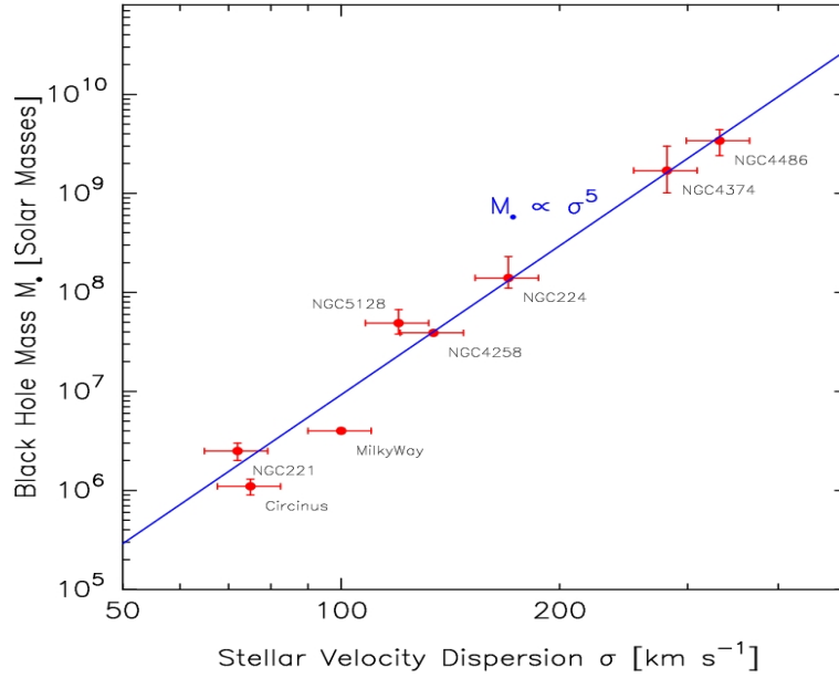
Σχήμα 4.2: Γραφική απεικόνιση της σχέσης M_\bullet - \sigma που βρίσκει εφαρμογή στους γαλαξίες. Οι μάζες των μελανών οπών των γαλαξιών που απεικονίζονται στο διάγραμμα έχουν υπολογιστεί με διάφορες παρατηρησιακές μεθόδους. Επέκταση του γραφήματος προς τα αριστερά, δηλαδή προς χαμηλότερες τιμές της ταχύτητας διασποράς \sigma , που παρατηρούνται σε ένα σφαιρωτό σμήνος, μπορεί να προσδιορίσει τη μάζα της IMBH που βρίσκεται στο κέντρο του.
