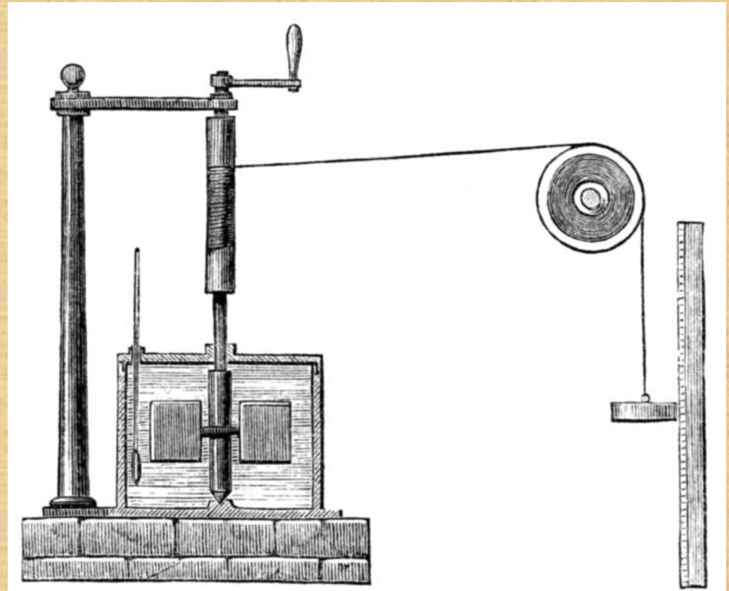
Πρωτότυπο ρεξοπλισμός του Joule, 1845
